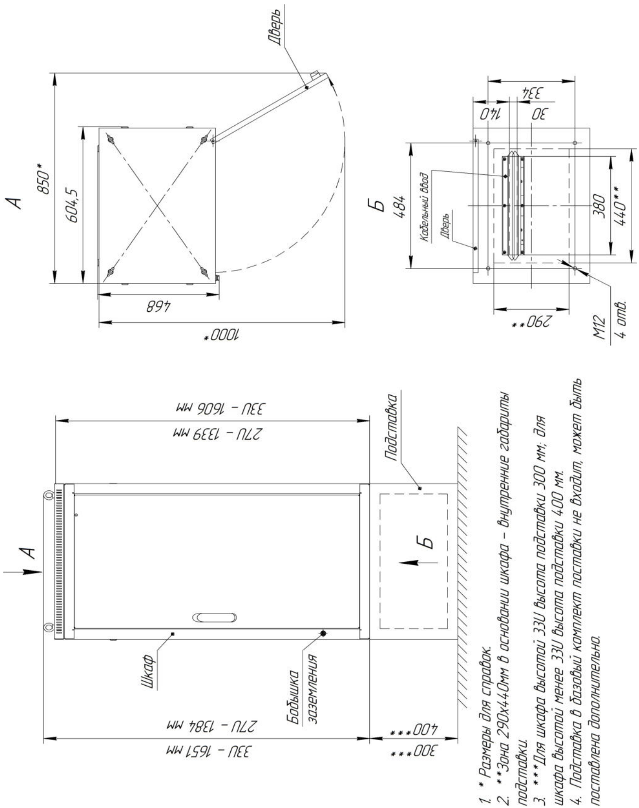
Рисунок П.1 – Габаритные и установочные размеры шкафа многоканального КМО на подставке (количество каналов до шести, исполнение У2)
