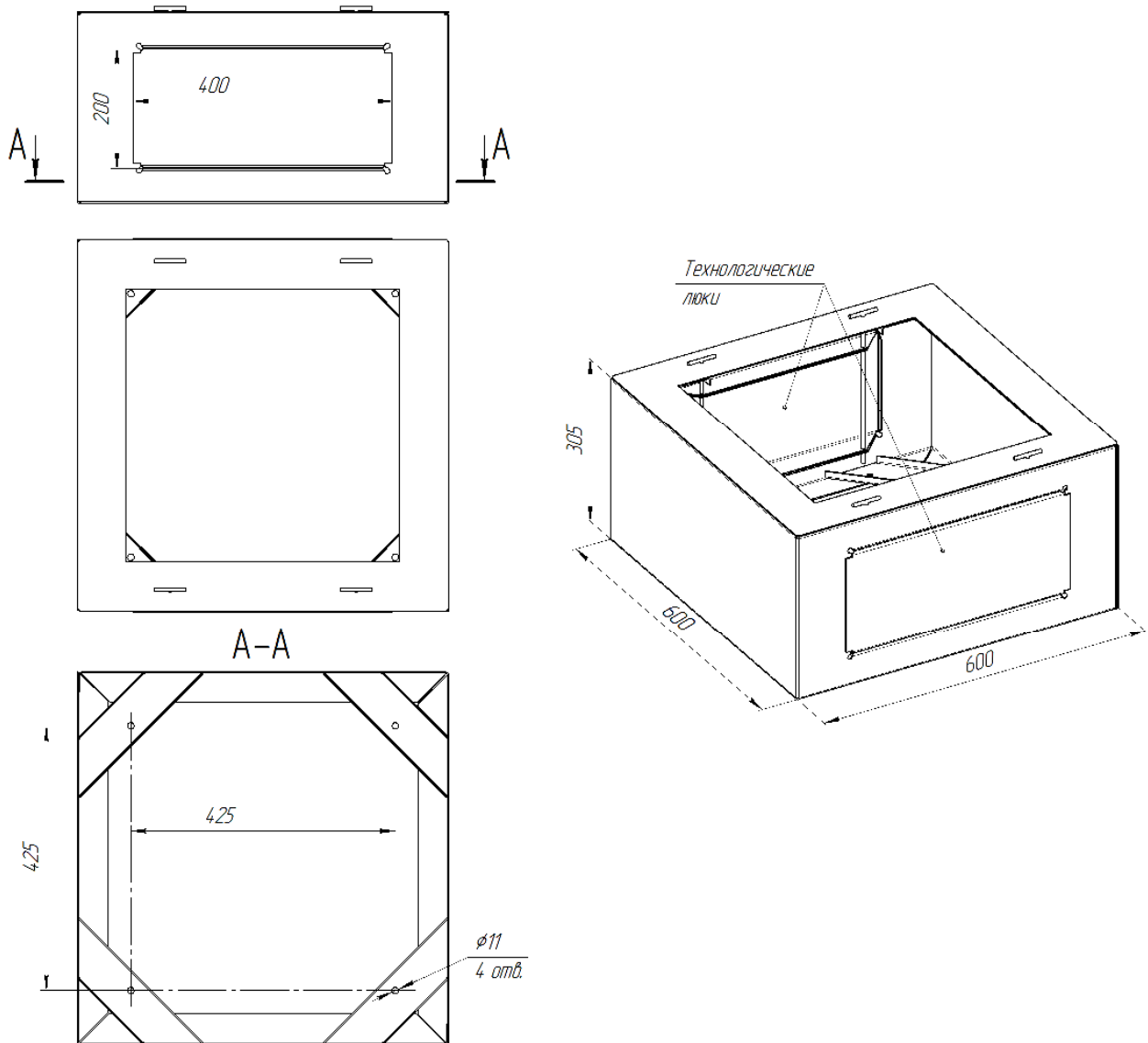
Рисунок П.5 – Подставка для шкафа исполнения У1
