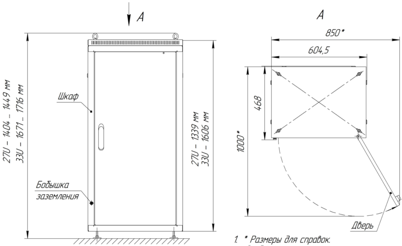
Рисунок П.2 – Габаритные и установочные размеры шкафа многоканального КМО на ножках (количество каналов до шести, исполнение У2)
