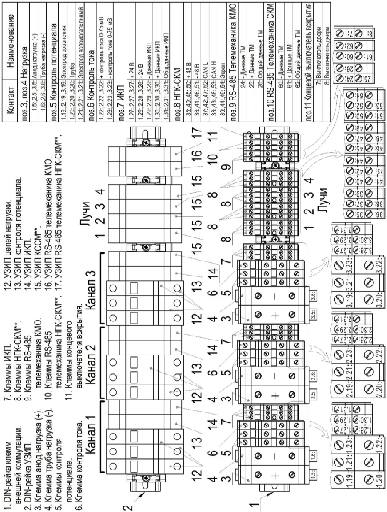
Рисунок К.3 – Расположение элементов на коммутационных DIN-рейках многоканального КМО с тремя каналами климатического исполнения У2 (лист 1)
