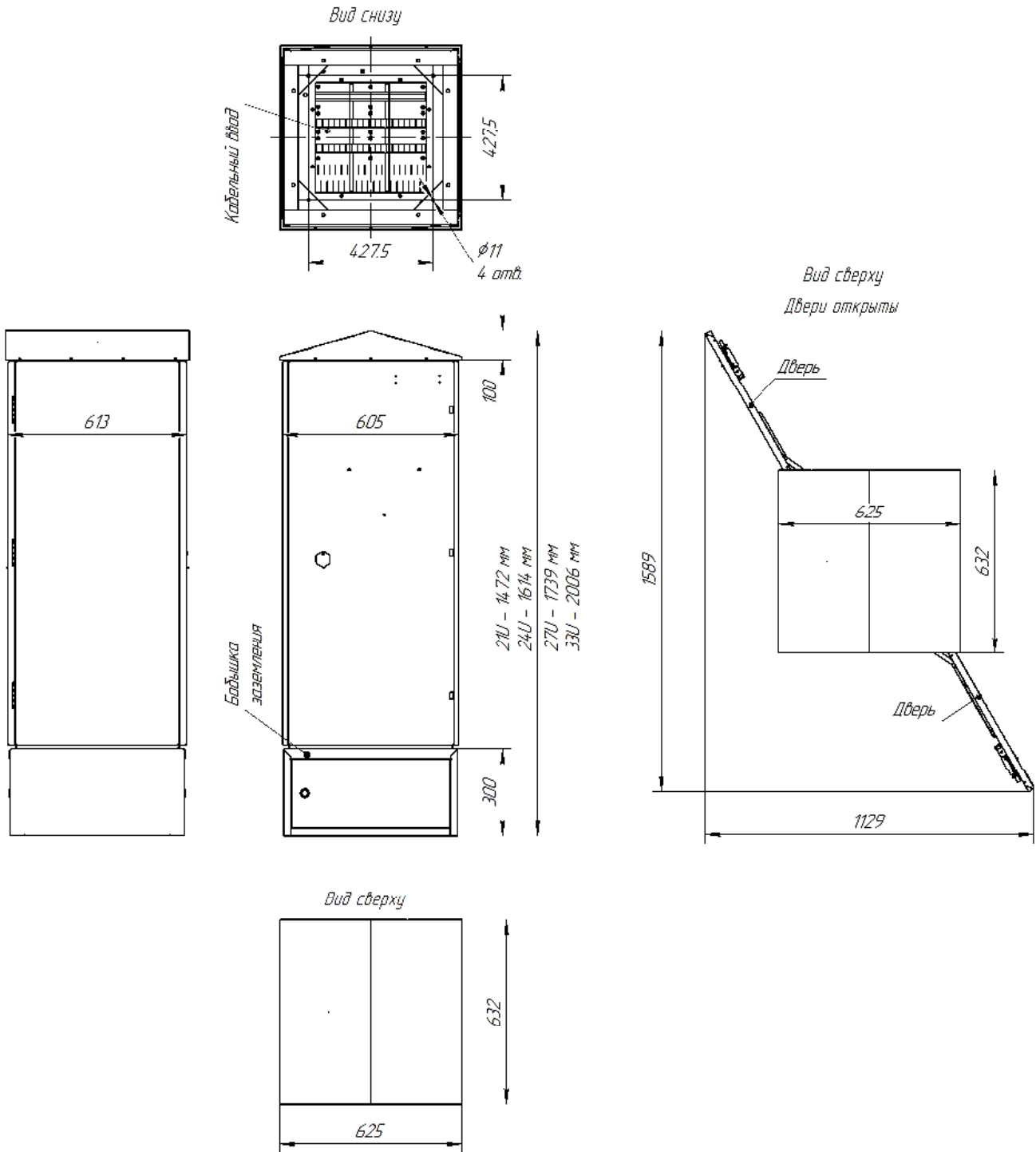
Рисунок П.3 – Габаритные и установочные размеры шкафа многоканального КМО (количество каналов до шести, исполнение У1)
