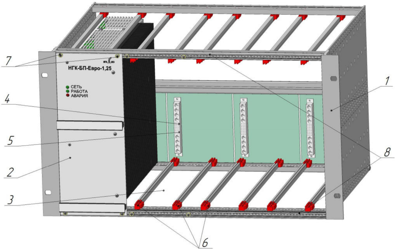
Рисунок Б.1 – Общий вид блочного каркаса модулей силовых НГК-БП-Евро-1,25(48)
